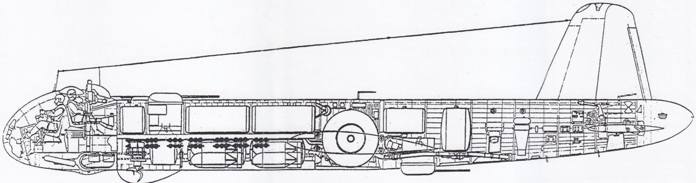
Компановочный чертеж фюзеляжа 140 B/R
