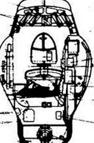
Schnitt E-F Schnitt E-F
