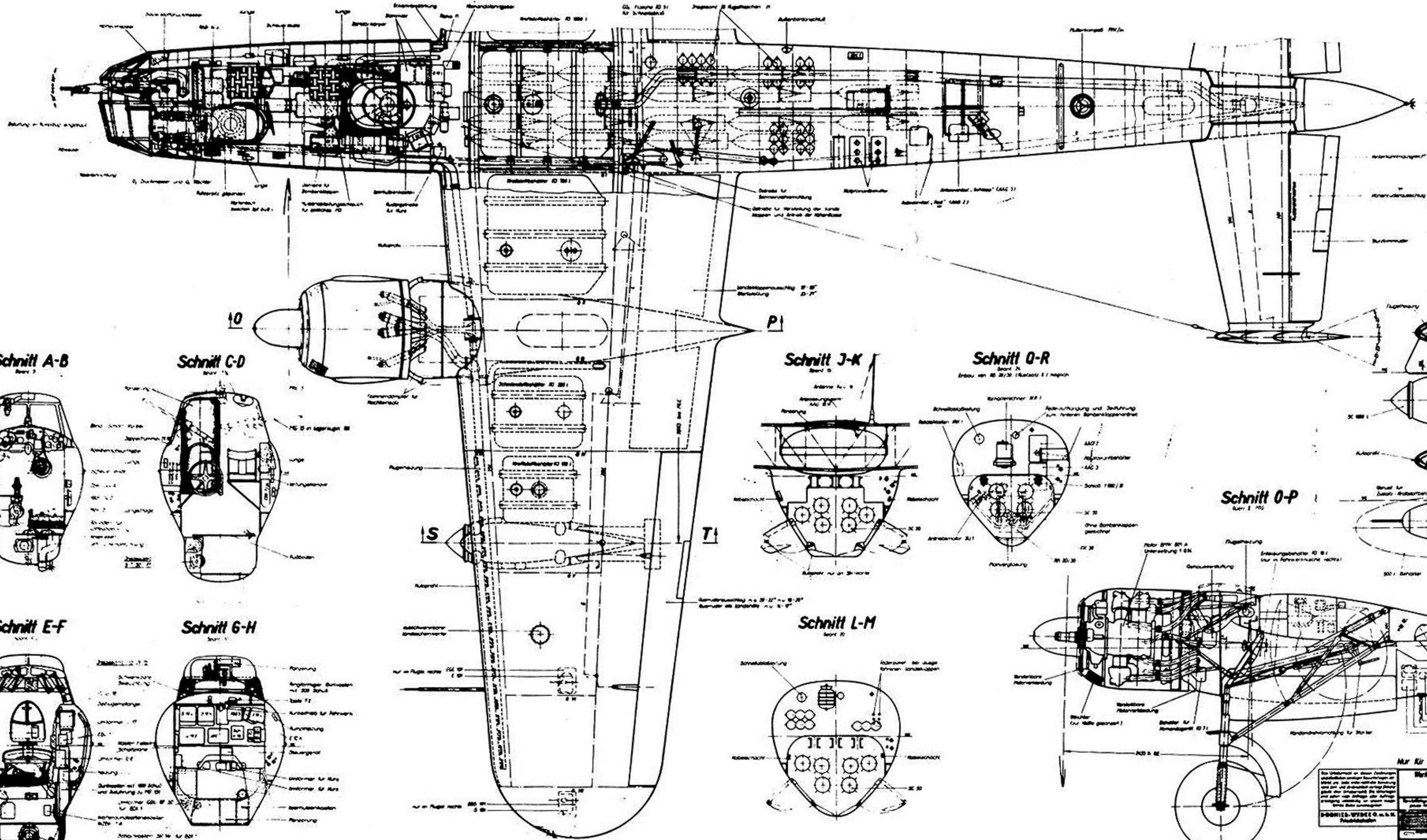
Schnitt S-T Schnitt S-T
