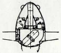
Schnitt E-F
