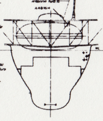
Schnitt L-M
