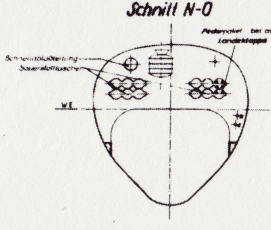
Schnitt N-O
