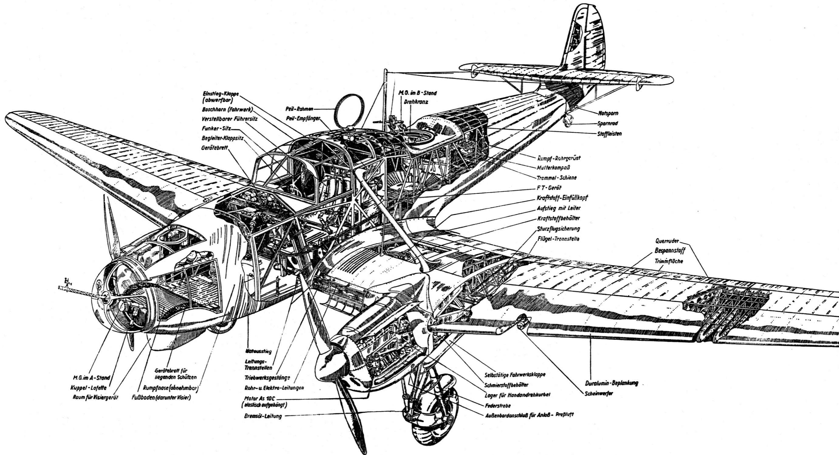
Militärisches Übungsflugzeug Fw 58 „Weihe“
