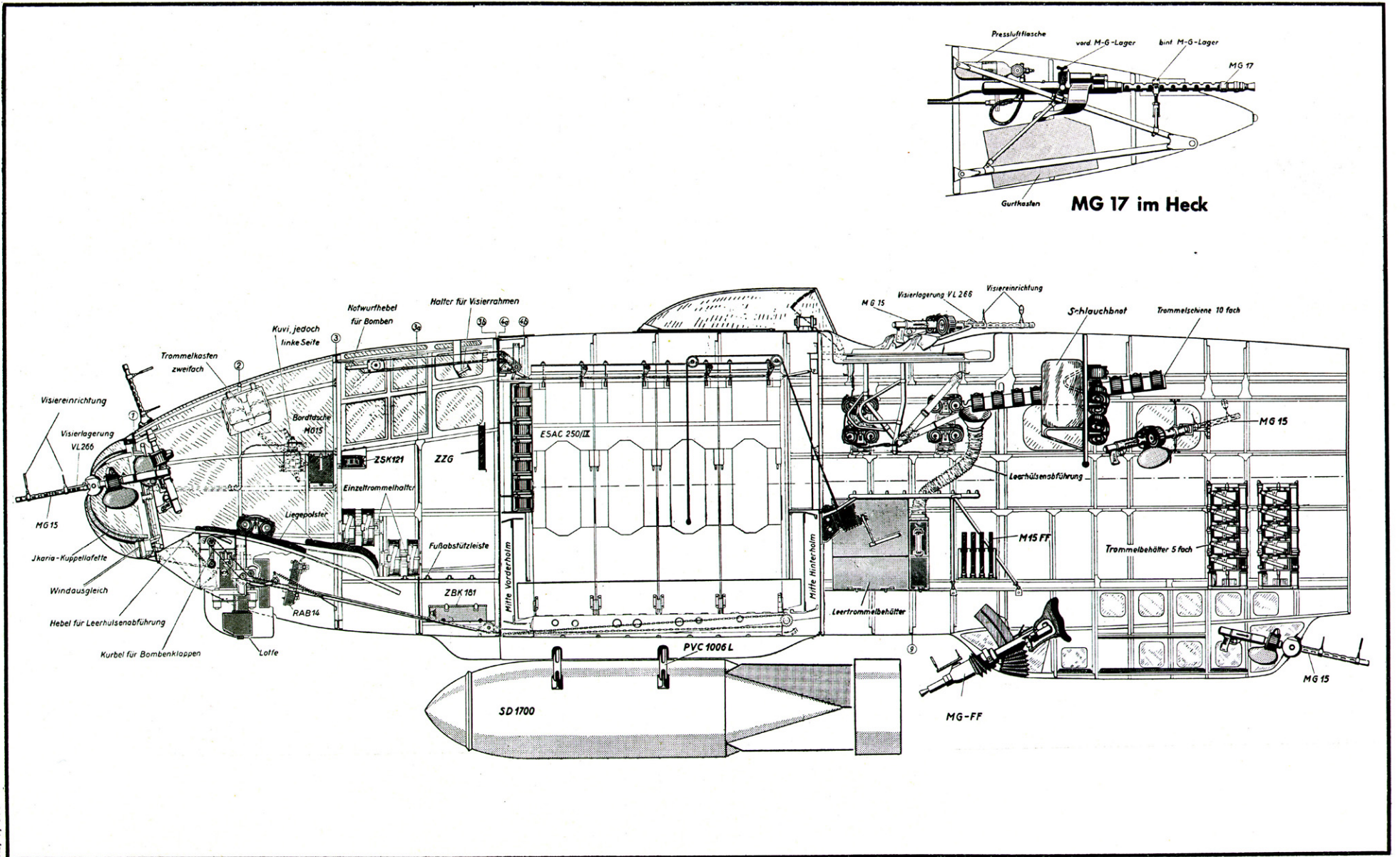
Gesamtübersicht der Bewaffnung He 111 H-5
