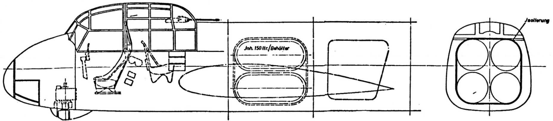
Ju88 S-1 Schnellbomber
