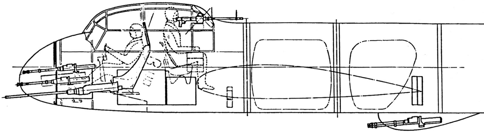
Ju88 C-5 Zerstörer
